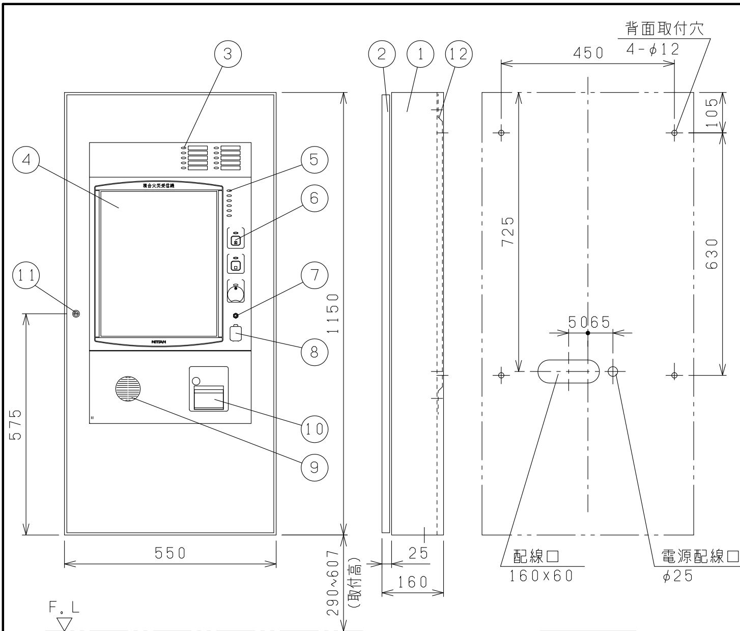
取付寸法図
